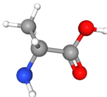
D-Alanine
